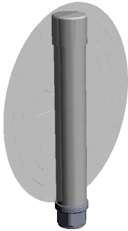
XZ-Plane Gain
