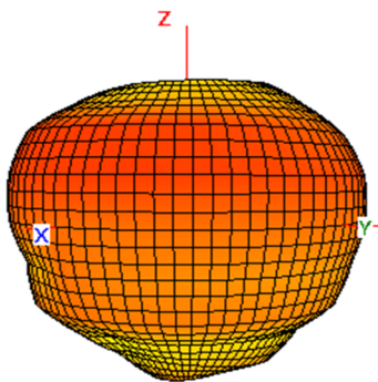
2400 MHz
