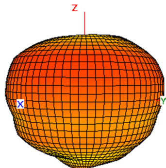
2450 MHz
